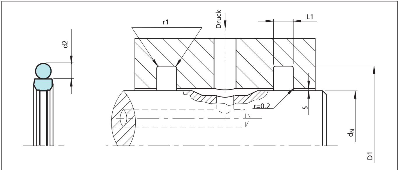
Bild 10 Einbauzeichnung
