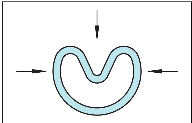
Bild 7 Nierenförmige Verformung des Dichtrings
