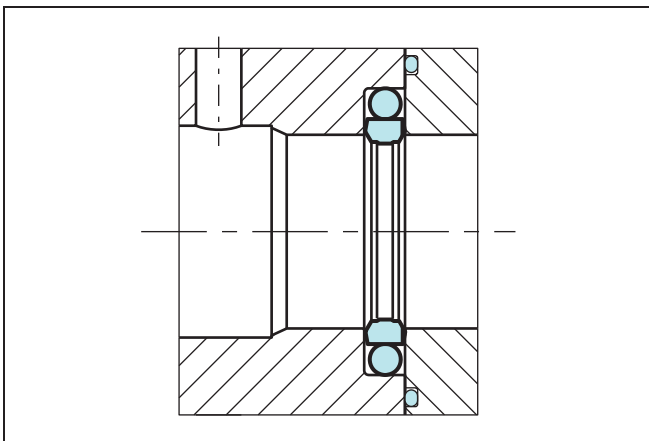
Bild 6 Einbau in eine geteilte Nut
