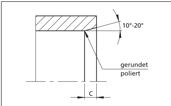
Bild 4 Einführungsschräge am Gehäuse
