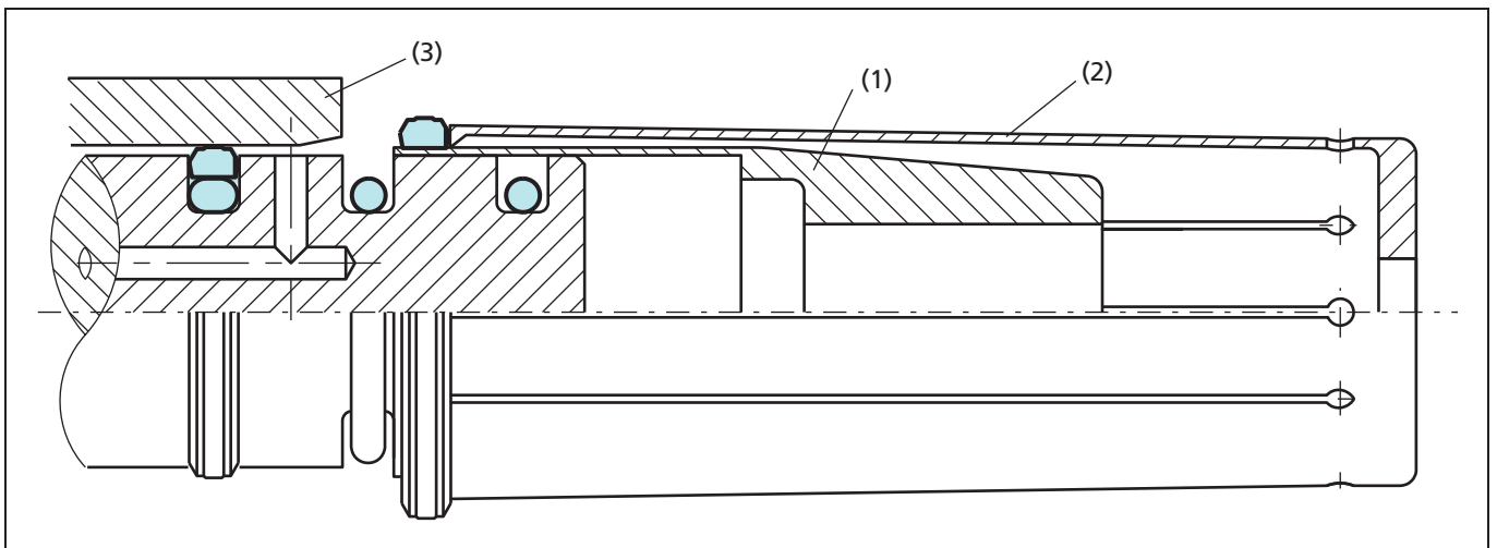
Bild 9 Aufdehnen des Zurcon® Roto Glyd Ring® S über die Montagehülse mittels einer Sprezhülse
