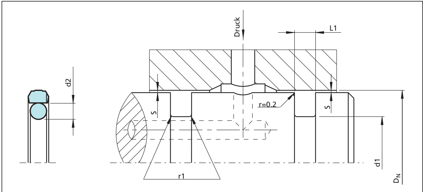
Bild 11 Einbauzeichnung
