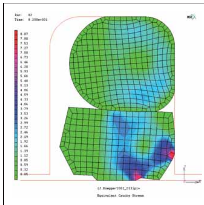
Bild 2 Zurcon® Roto Glyd Ring® S - Finite Element Analysis (FEA)
