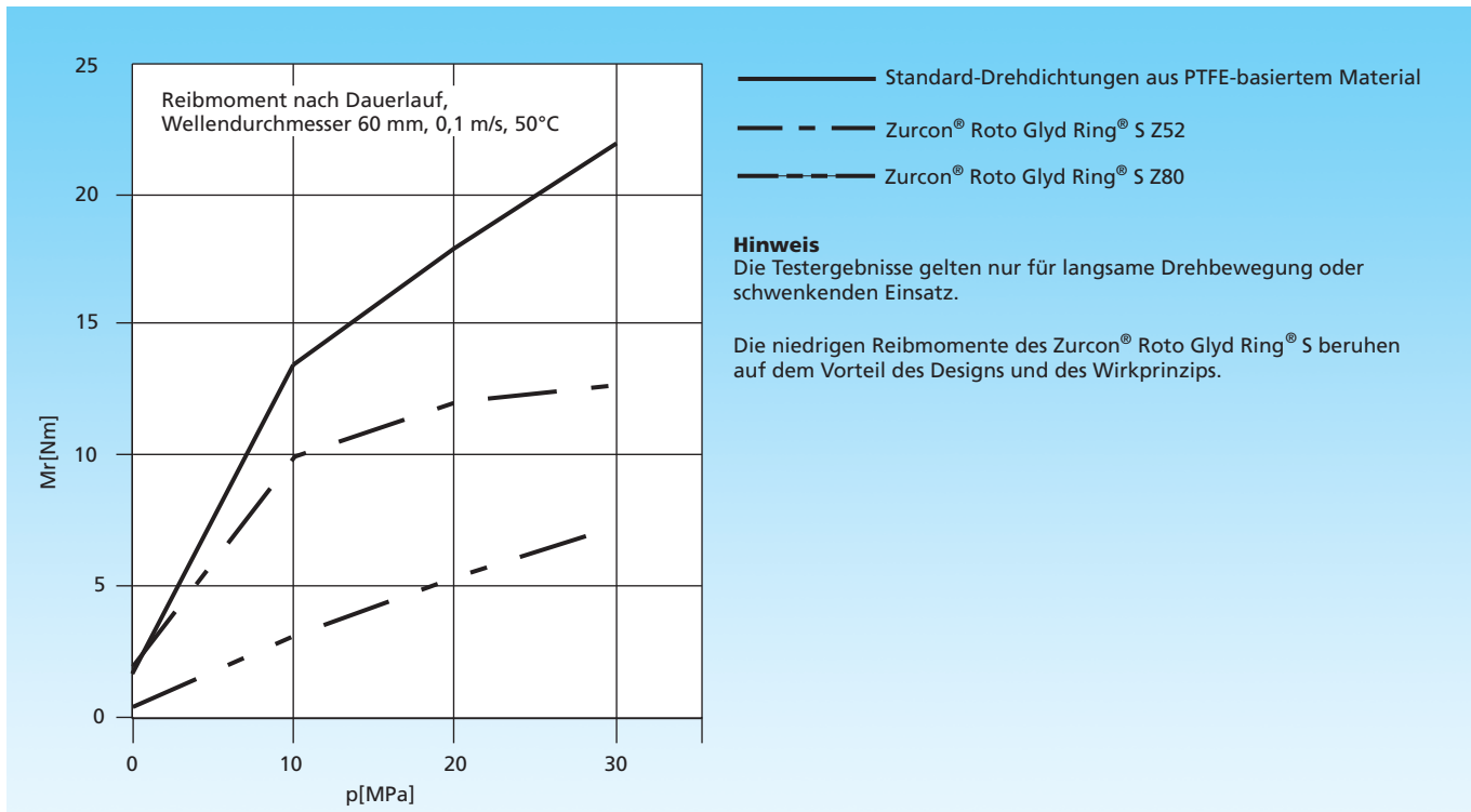
Bild 3 Reibmomente der Dichtungen nach Test
