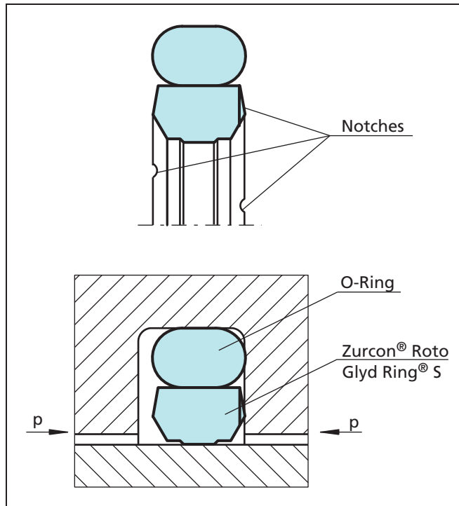
Bild 1 Zurcon® Roto Glyd Ring® S
