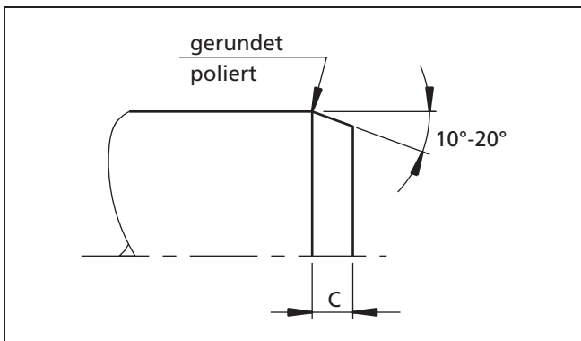
Bild 5 Einführungsschräge an der Welle
